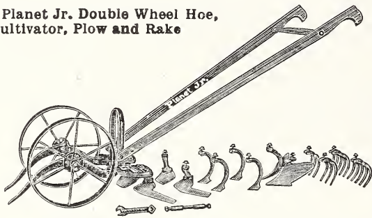
No. 8 Planet Jr. Horse Hoe
